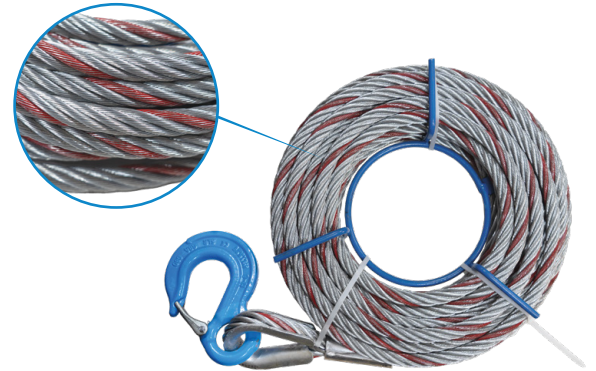
Cable de acero: 20 m (estándar) Opcional: longitud según requerimiento
